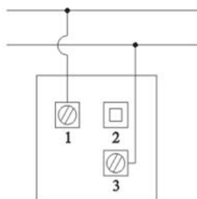
Hz meter
