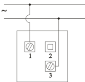
交流电压表
