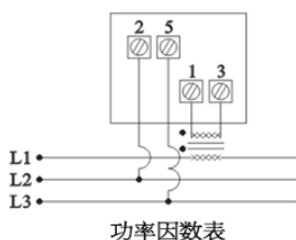
功率因数表
