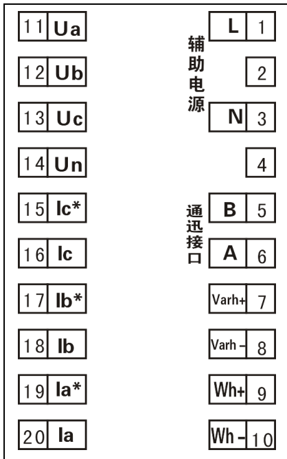
JYS-2S4端子接线：
