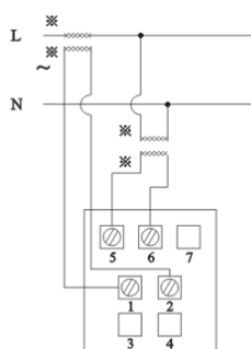
单相功率表 (配电流和电压互感器)
