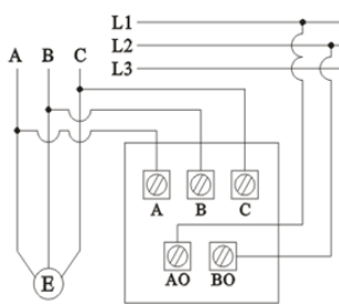
三相同步表
